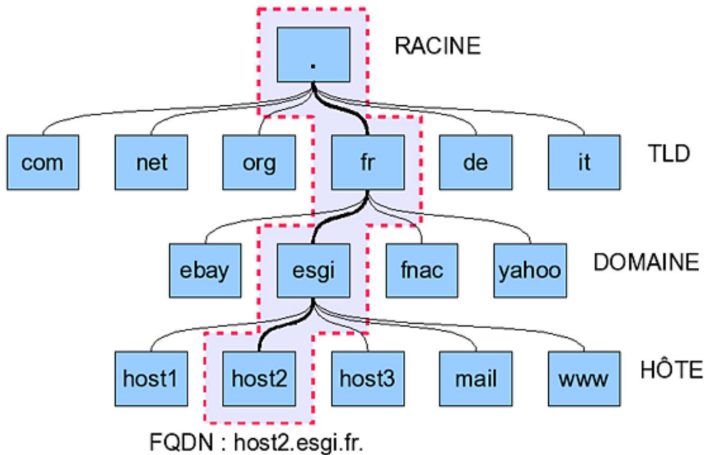
Représentation d'une arborescence DNS
